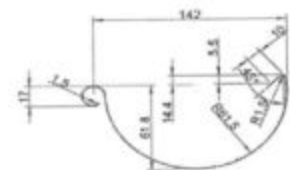
Сечение желоба
